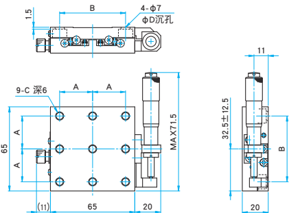
TSD-651SZ25-M6/651SZ25UU
