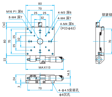
TAM-802C 内六角螺栓 M4×8...4个
