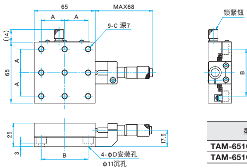
TAM-651C-M6/651CUU 内六角螺栓 M6×8...4个 (M6) 内六角螺栓 1/4-20UNC×3/8...4个 (UU)
