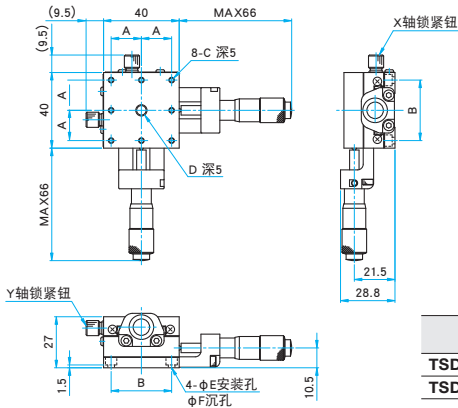
TSD-402C/402CUU 内六角螺栓 M3×6...4个 内六角螺栓 6-32UNC×3/16...4个 (UU)
